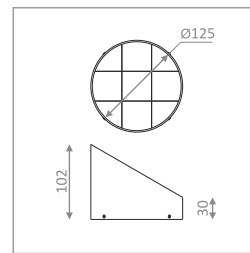
PHIL53 SK VIGO LED anti-glare cover-diagonal osłona antyolśnieniowa skośna black • czarny A8980002
