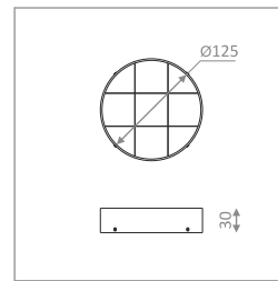
PHIL53 SK VIGO LED anti-glare cover-straight osłona antyolśnieniowa prosta black • czarny A8990002
