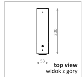
connector I 200 łącznik I 200
