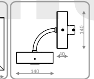
F - 74790020 anod.
