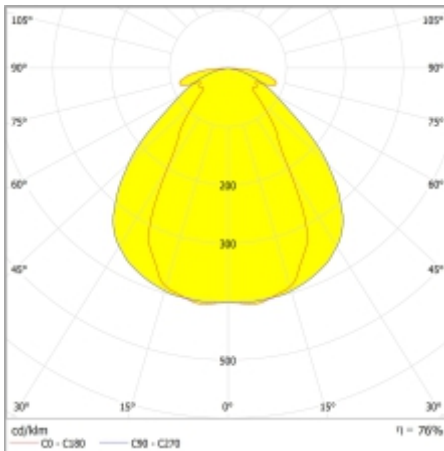
cover PH/LO/SM NARROW, light curve • klosz PH/LO/SM NARROW, krzywa światłości
