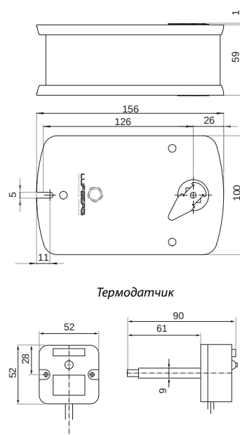
РАЗМЕРЫ (мм)
