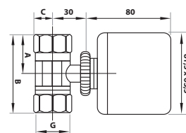
РАЗМЕРЫ (ММ)
