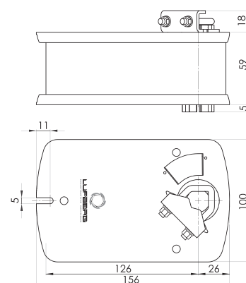
РАЗМЕРЫ (мм)
