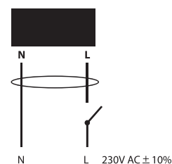
ЭЛЕКТРИЧЕСКОЕ ПОДКЛЮЧЕНИЕ
