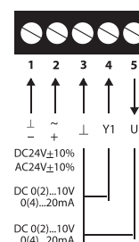
Пропорциональное 24 В
