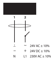
ЭЛЕКТРИЧЕСКОЕ ПОДКЛЮЧЕНИЕ
