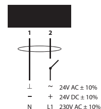
ЭЛЕКТРИЧЕСКОЕ ПОДКЛЮЧЕНИЕ
