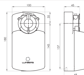
РАЗМЕРЫ (мм)
