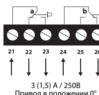
Вспомогательные переключатели
