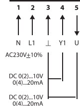
Пропорциональное 230 В
