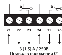
Вспомогательные переключатели
