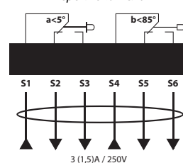
Вспомогательные переключатели
