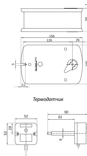
РАЗМЕРЫ (мм)
