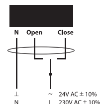
ЭЛЕКТРИЧЕСКОЕ ПОДКЛЮЧЕНИЕ
