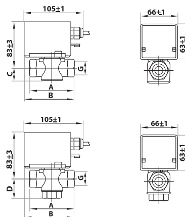
ГАБАРИТНЫЕ РАЗМЕРЫ (ММ)
