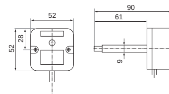
Термодатчик
