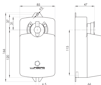
РАЗМЕРЫ (мм)
