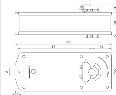
РАЗМЕРЫ (ММ)
