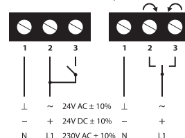
2-х/3-х позиционное
