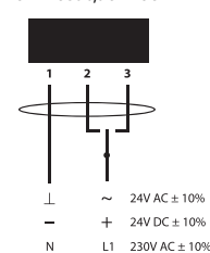
3-х позиционное
