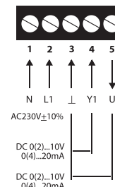
Пропорциональное 230 В
