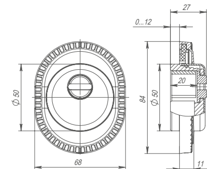
Броненакладка ET/ATC-Protector 1CL-25
