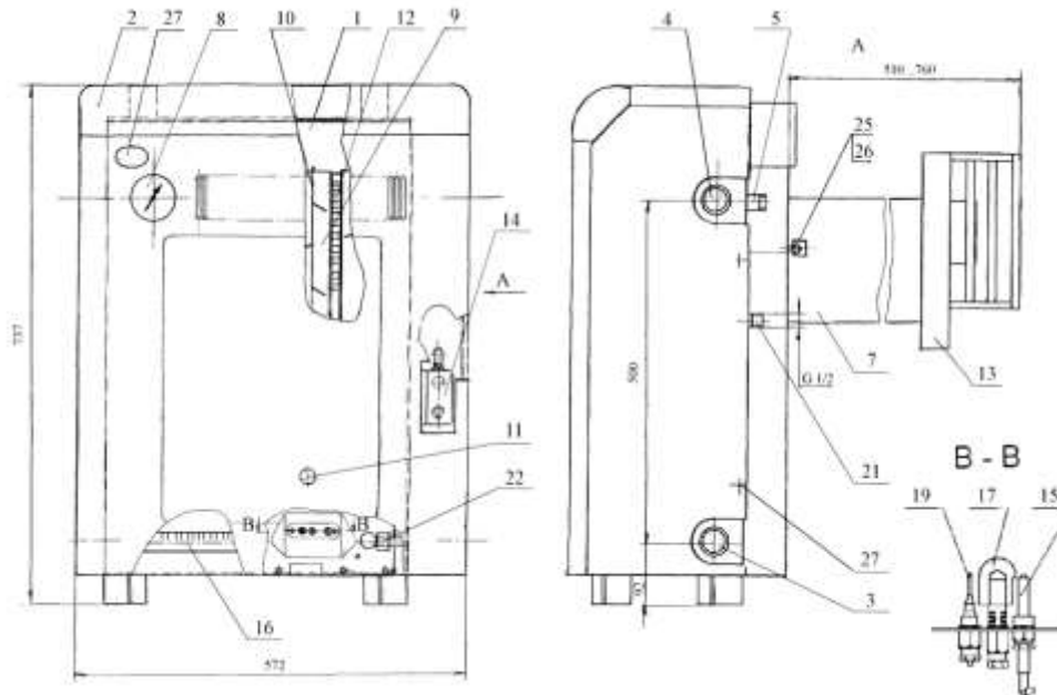
Рис. 1 – Будова апарата
