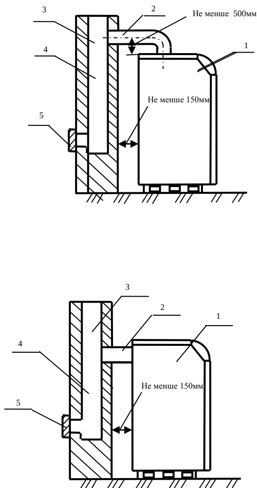
Рис.2.1 Схема встановлення апарата 1-апарат; 2-з'єднувальний патрубок ; 3-димохід; 4- кишеня; 5- дверці для чистки димохода.
