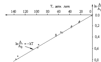
Рис. 15. Линейная зависимость \ln(A/A_0) от возраста T . Кружочки — значения \ln(A/A_0) , вычисленные авторами [Осипишин]. Крестики — те же значения по данным А. Б. Ронова и др.
