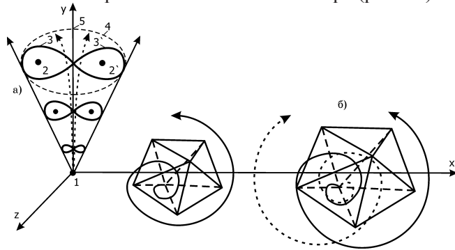
Рис. 12. Структура поливихревой системы
