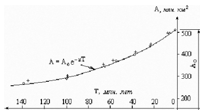
Рис. 14. Ход ускоренного формирования площадей океанической коры. Кружочками обозначены значения площадей A , подсчитанные на начало геологических эпох. Крестики — данные А. Б. Ронова с соавторами
