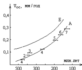
Рис. 16. Изменение во времени данных по скоростям накопления осадков и их погружения в рифтогенных прогибах Западно-Арктического шельфа (А), и скорости прогибания геосинклинальных прогибов (Б) по Л. И. Салопу, 1973 г.
