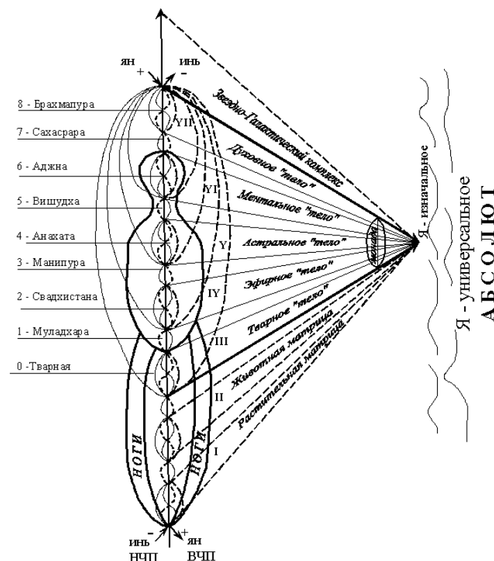
Рис. 18. Структура энергоинформационного каркаса человека (ЭИКЧ)
