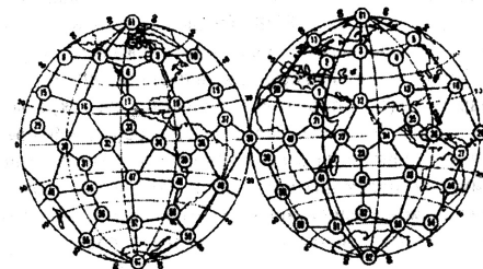
Рис. 11. Икосаэдро-додекаэдрическая решетка разломов Земли
