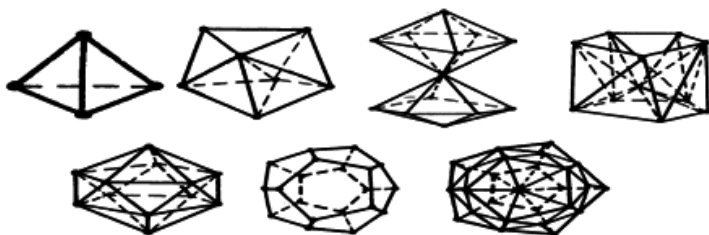
Рис. 10. Структурные модели стационарного состояния систем
