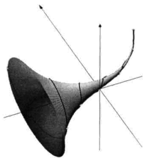
Рис. 6. Поверхность «Золотой шофар»
