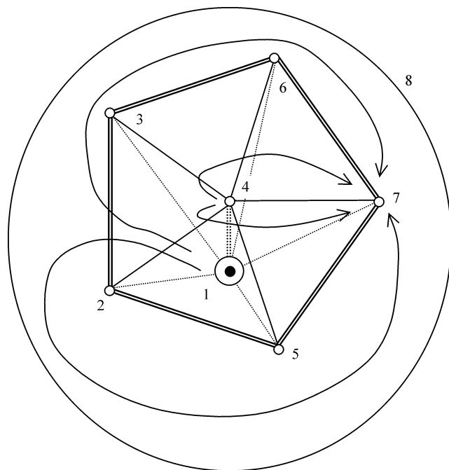
Рис. 8. Пентатетраэдр как структурно-функциональная модель системы
