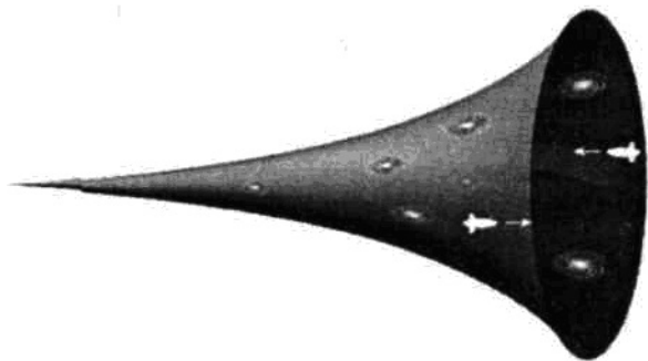
Рис. 5. Генетическая форма Вселенной
