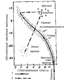
Рис. 17. Расположение звезд и планет на диаграмме Герцшпрунга-Рессела: 1 - постепенные переходы звезд от одного класса к другому; 2 - спонтанные переходы по мере развития звезд, вызванные нестационарными процессами
