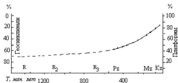
Рис. 13. Ускоренное становление земной коры континентов по Н. С. Шатскому
