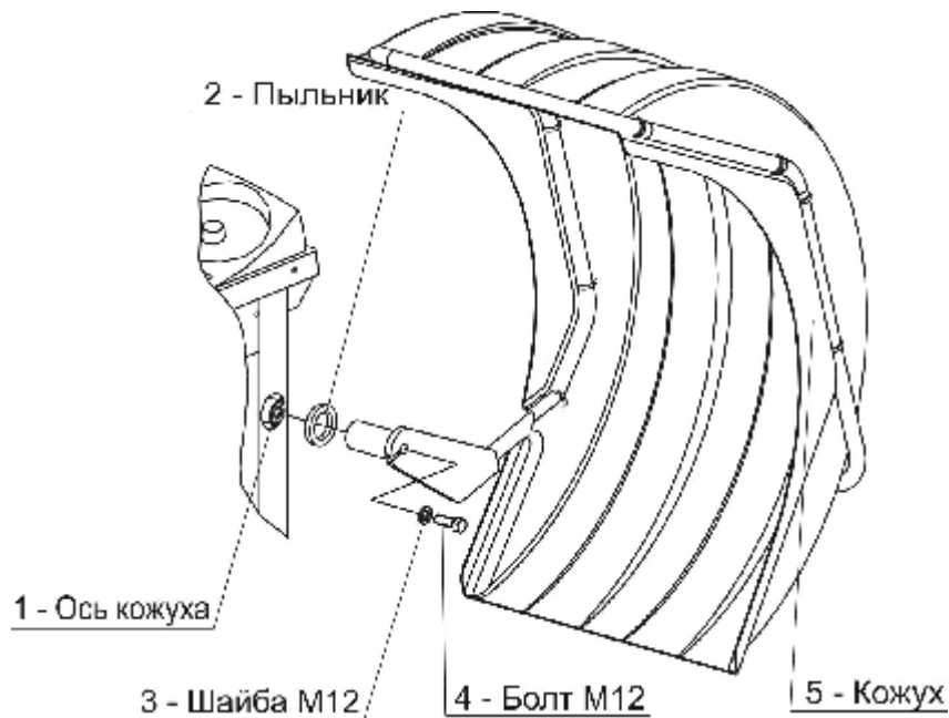
г – установка кожуха
