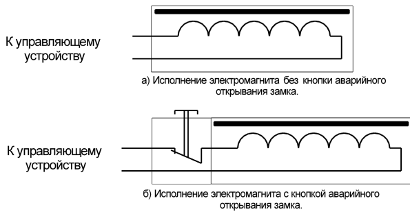
Рис. 3. Схема электрическая принципиальная
