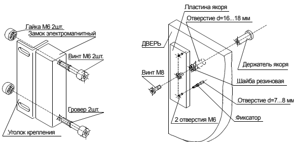
Рис. 1. Вариант крепления электромагнитного замка к раме двери.
