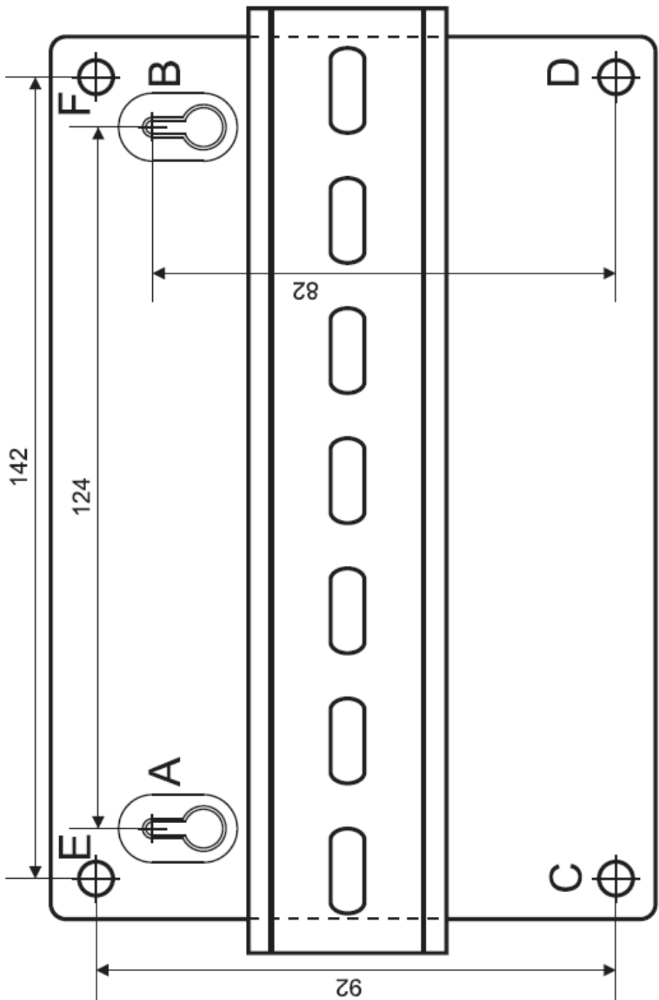
Рисунок 17. Шаблон для монтажа
