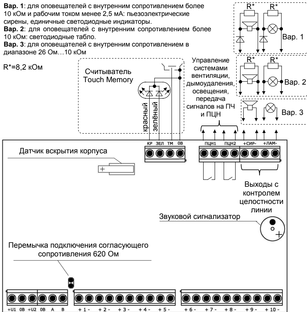
Рисунок 4. Схема внешних соединений прибора
