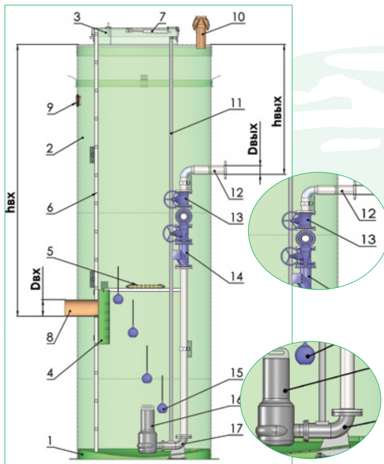
Схема КНС с погружными насосами
