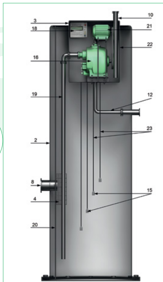
Схема КНС с самовсасывающими насосами
