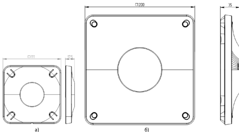
Рисунок 1 – Габаритные размеры светодиодного светильника серии Public:
